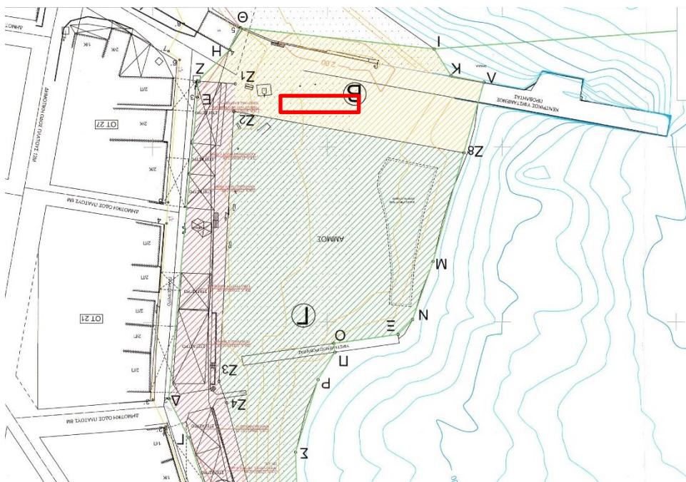
Εικόνα 1: Απόσπασμα από Τοπογραφικό Σχέδιο Λιμένα Ουρανούπολης με απεικόνιση του σημείου στο οποίο προβλέπεται η τοποθέτηση της Κατασκευής Χώρου Εκδοτηρίων και Στάσης Αναμονής Επιβατών.
